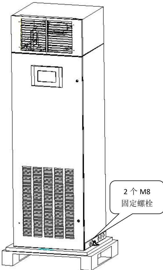
图 2.1.3 底板固定螺栓
