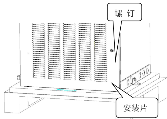
图 2.1.4 拆除安装片
