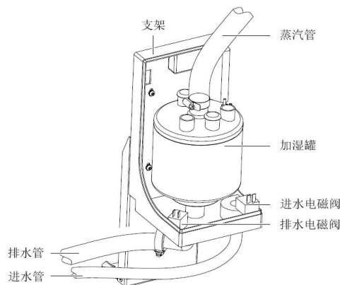
图 5.2.5 电极加湿器示意图
